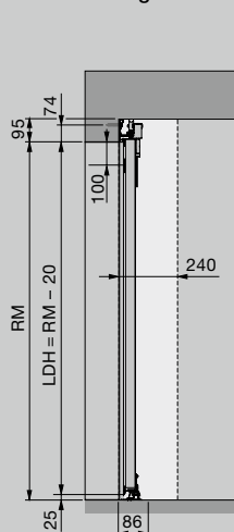
Wandmontage als schuifdeur
