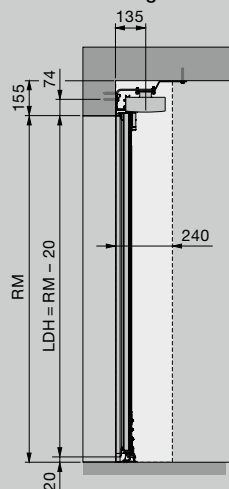
Plafondmontage B als schuifdeur
