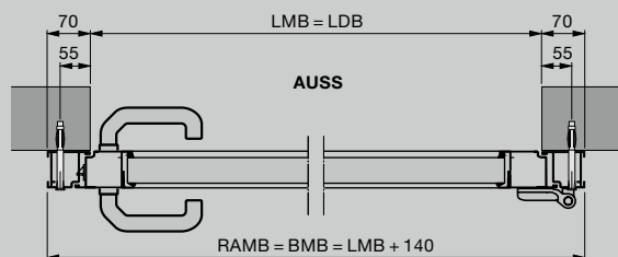
Zijdeur met aluminium blokkozijn Inbouw achter de opening
