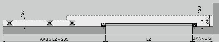
Plafondmontage B als schuifdeur (doorsnede van de vloerrail)
