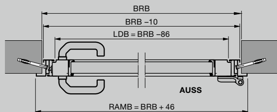
Zijdeur met hoekkozijn Inbouw voor de opening
