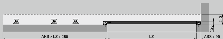
Wandmontage als schuifdeur (doorsnede van de vloerrail)
