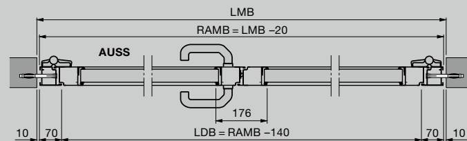
2-vleugelige zijdeur met aluminium blokkozijn Inbouw in de opening
