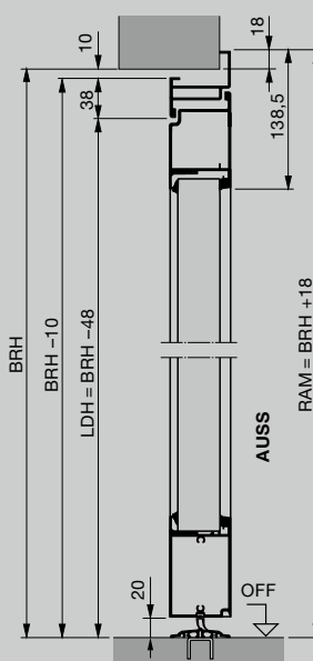
Zijdeur met aluminium hoekkozijn Buitenaanslag
