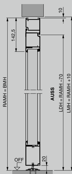
Zijdeur met aluminium blokkozijn Inbouw in de opening
