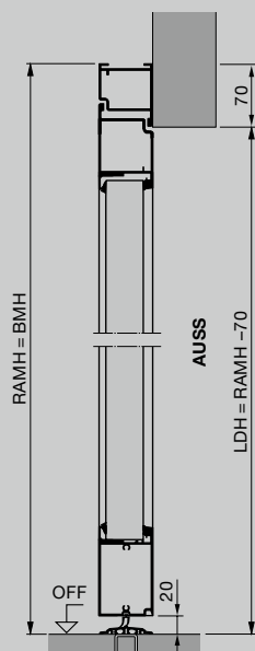
Zijdeur met aluminium blokkozijn Inbouw achter de opening
