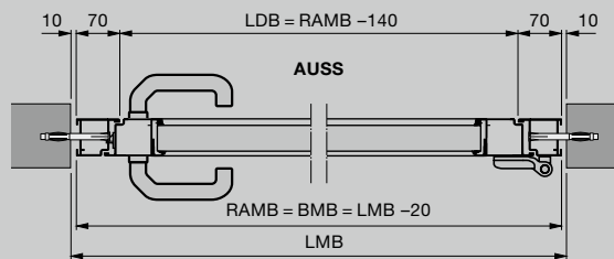
Zijdeur met aluminium blokkozijn Inbouw in de opening
