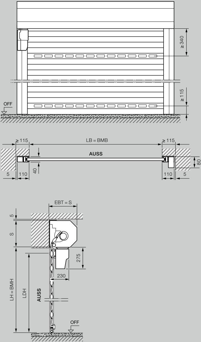
Maatbereik binnen- en buitenroldeur
