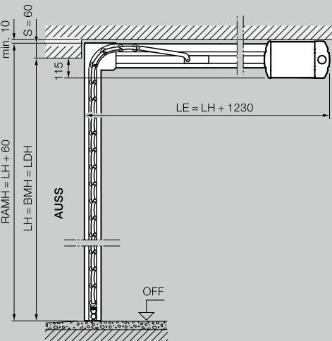
Maatbereik RollMatic OD-garagedeur*
